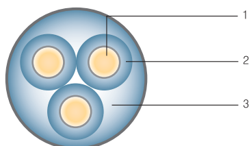
1. 도 체 1. Conductor 2. 절연체 2. Insulation 3. 시 스 3. Sheath
